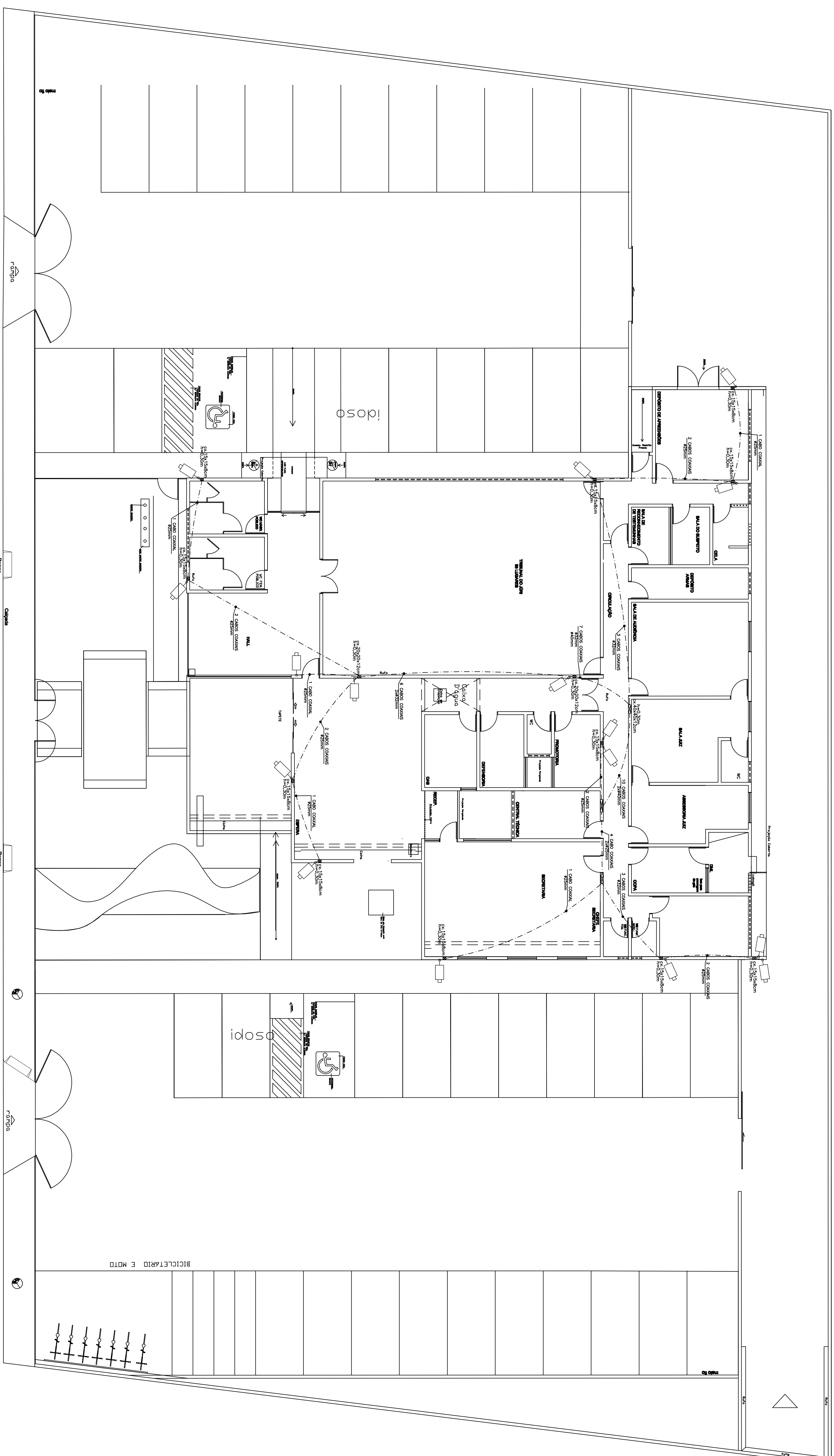
PLANTA BAIXA - CFTV Esc-----1/100
